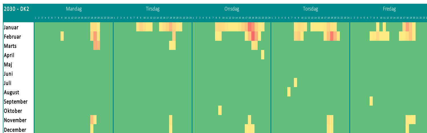
Figur 18 Fordeling af effektminutter på måned, ugedag og time i døgnet (1-24) i 2030 i Østdanmark. Jo rødere nuancer, jo større vurderes risikoen for manglende effekttilstrækkelighed. Lørdag og søndag er udeladt, da de kun er grønne på tværs af måneder og time i døgnet.
