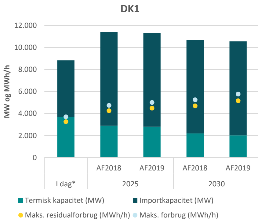
Figur 13 Udvikling for Vestdanmark i AF2018 og AF2019. Residualforbrug er givet ved forbruget fratrasket den indenlandske produktion fra vind og sol på timeniveau. Maks. residualforbrug og maks. forbrug er baseret på output fra Energinets BID-model. *Kapaciteter for i dag er baseret på 2020-værdier fra AF2019, mens maks. residualforbrug og maks. forbrug er baseret på 2019 observerede værdier.
