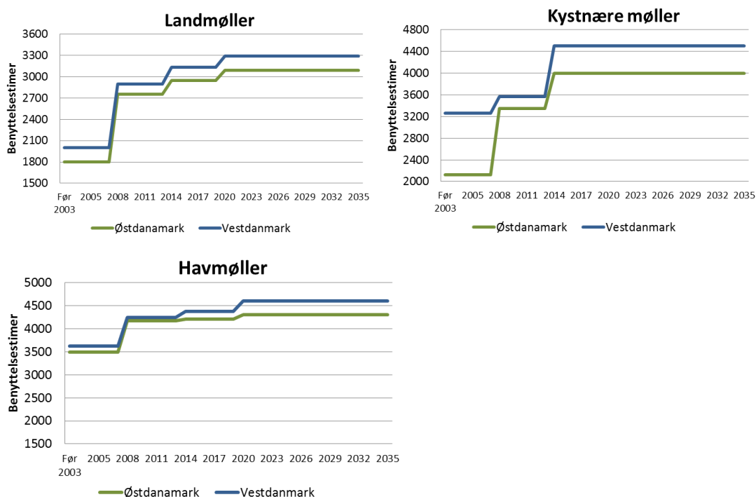
Figur 2 Benyttelsestider for vindkraft.
