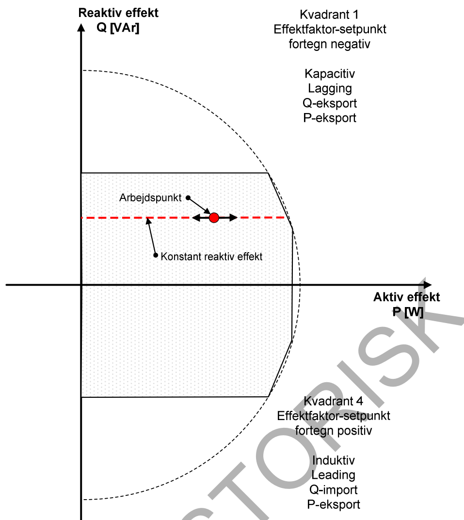
Figur 11 Reguleringsfunktioner for reaktiv effekt for et solcelleanlæg.
