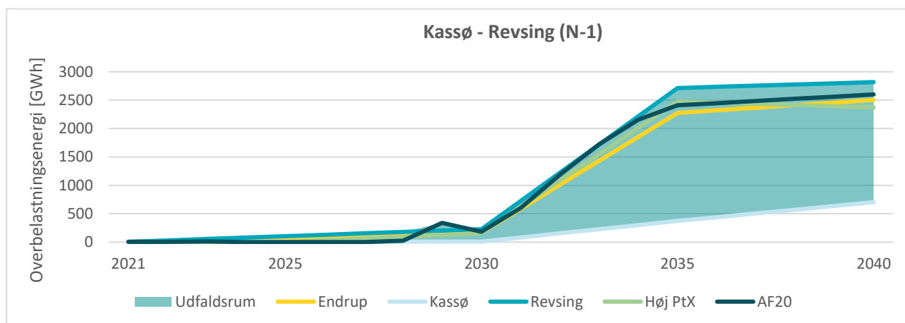
Figur 36 Overbelastningsenergi i 400 kV-forbindelsen Kassø-Revsing under hensyntagen til N-1. I AF20-scenariet er energiøen forudsat tilsluttet delt mellem Revsing og Tjele og i "Kassø", "Endrup" og "Revsing" er den fulde kapacitet tilsluttet i de stationer. For AF20 er resultaterne interpoleret mellem 2035 og 2040.
