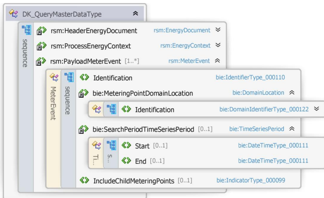
Figur 3434 - Klassediagram for forespørg om stamdata
