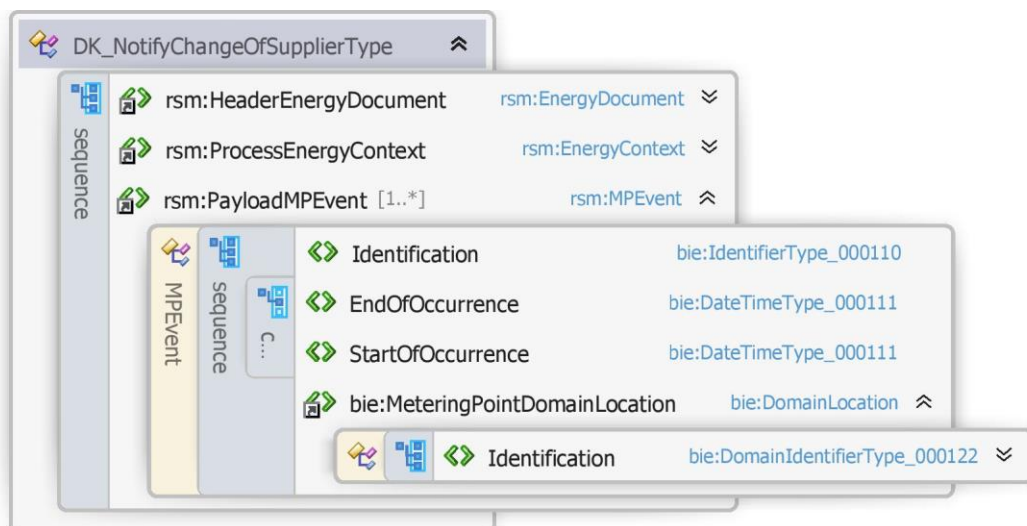
Figur 2626 - Klassesdiagram for Notifikation om skift af elleverandør
