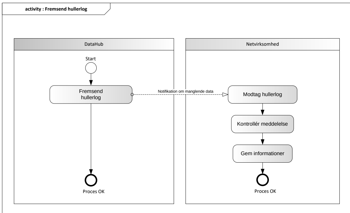
Figur 6969 - Aktivitetsdiagram for Fremsend hullerlog
