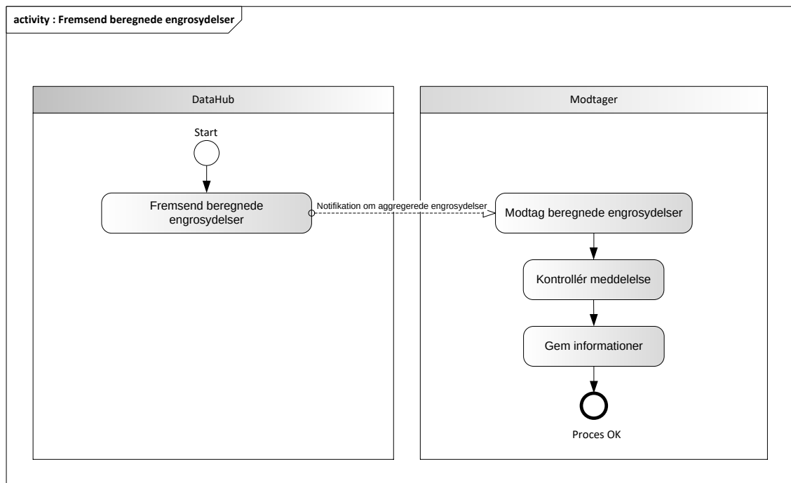
Figur 7272 - Aktivitetsdiagram for Fremsend beregnede engrosydeler
