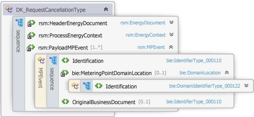
Figur 9292 - Klassediagram for Annullering af anmodning
