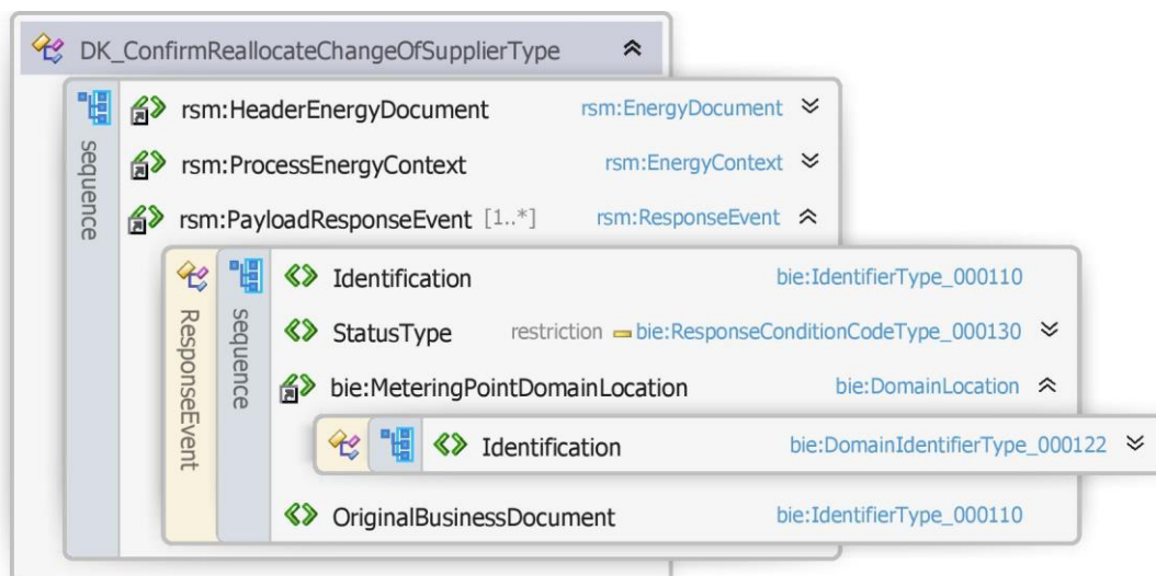
Figur 2222 - Klassesdiagram for Godkend tilbageføring af elleverandør
