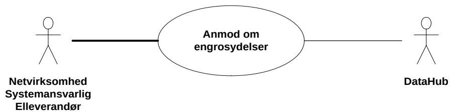
Figur 6464 - Use Case Diagram for anmod om engrosydelse
