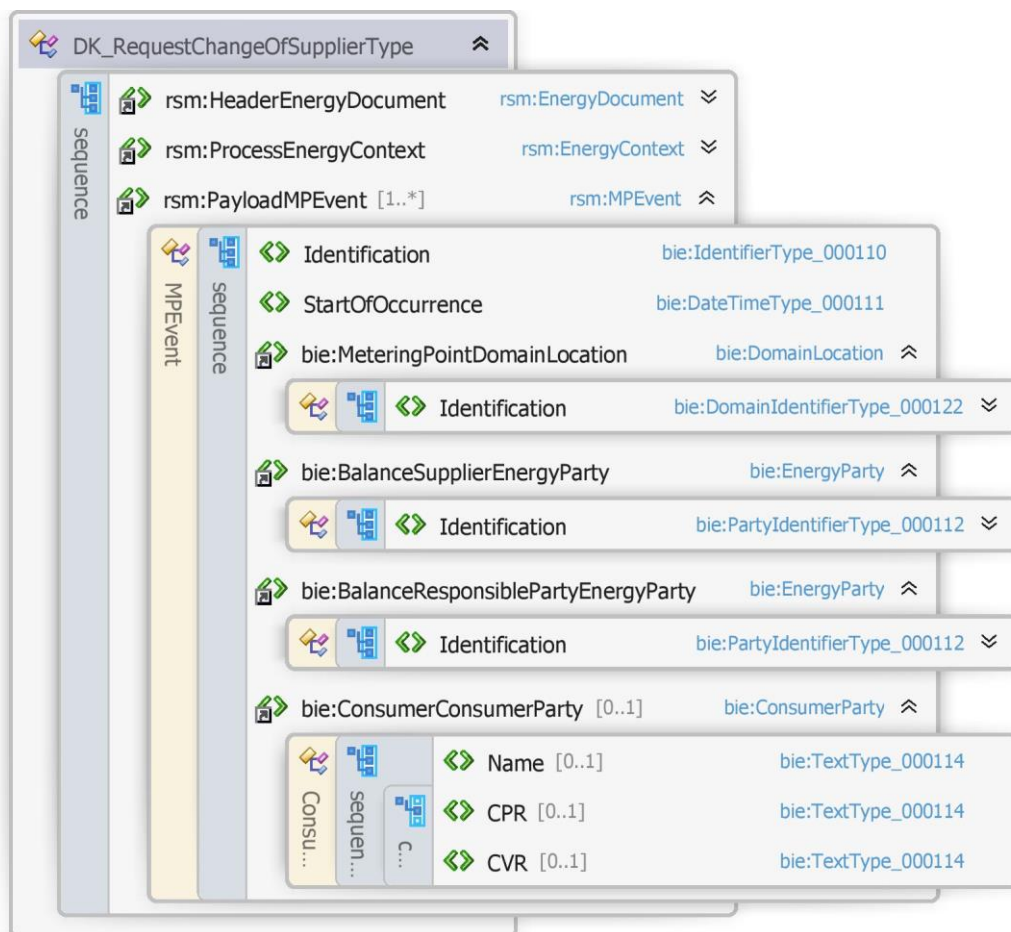
Figur 1111 - Klassediagram for Anmod start af leverance
