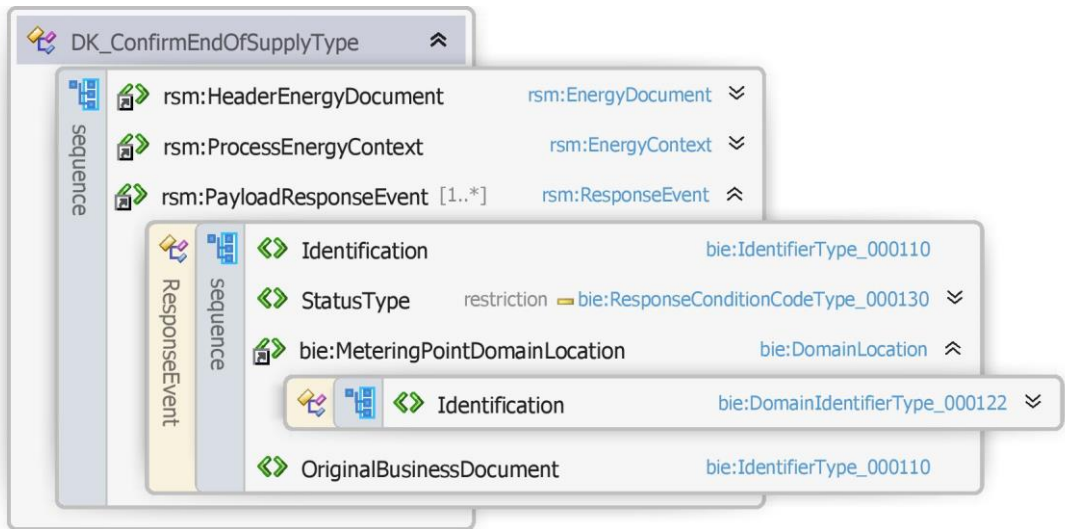
Figur 3030 - Klassediagram for Godkend leveranceophør
