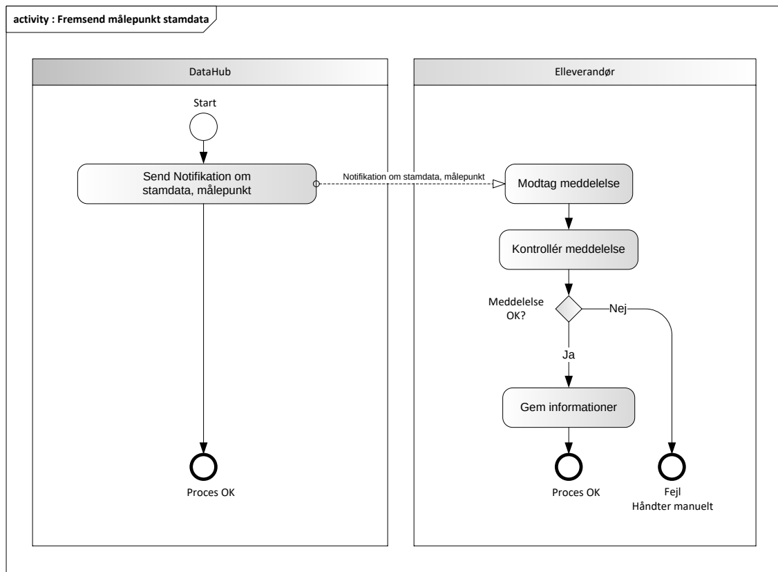
Figur 8585 - Aktivitetsdiagram for Fremsend målepunkt stamdata
