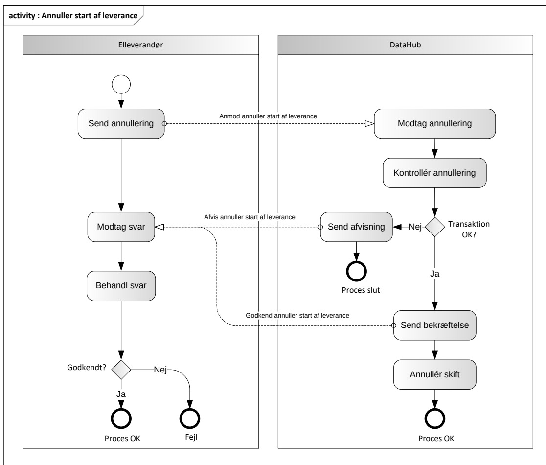
Figur 1515 - Aktivitetsdiagram for Annuller start af leverance
