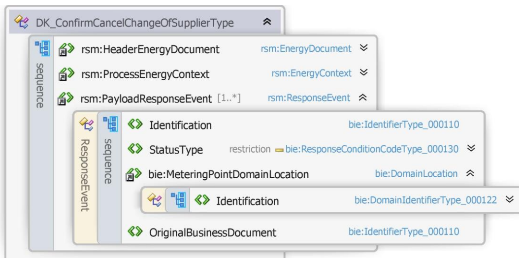
Figur 1717 - Klassediagram for Godkend annuller af start af leverance
