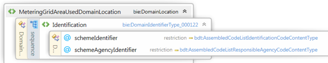
Figur 55 - XML Schema, Navn på type
