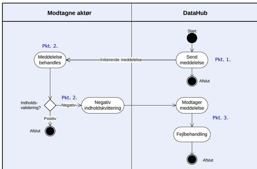
Figur 142142: Generisk kvitteringsflow – DataHub sender en meddelelse mod aktøren
