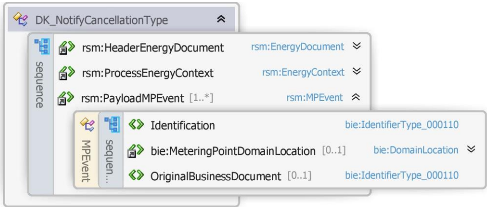
Figur 9797 - Klassesdiagram for Notifikation om annullering
