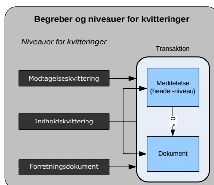
Figur 140140: Begreber og niveauer for kvitteringer
