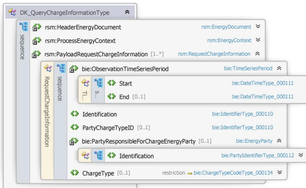
Figur 132132 - Klassediagram for Forespørg på prisliste
