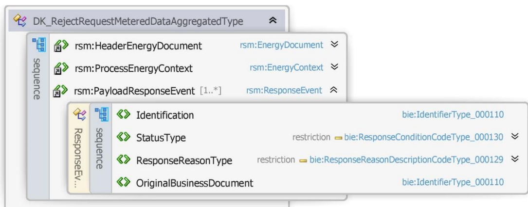
Figur 6363 - Klassediagram for Afvis anmod om aggregerede måldata
