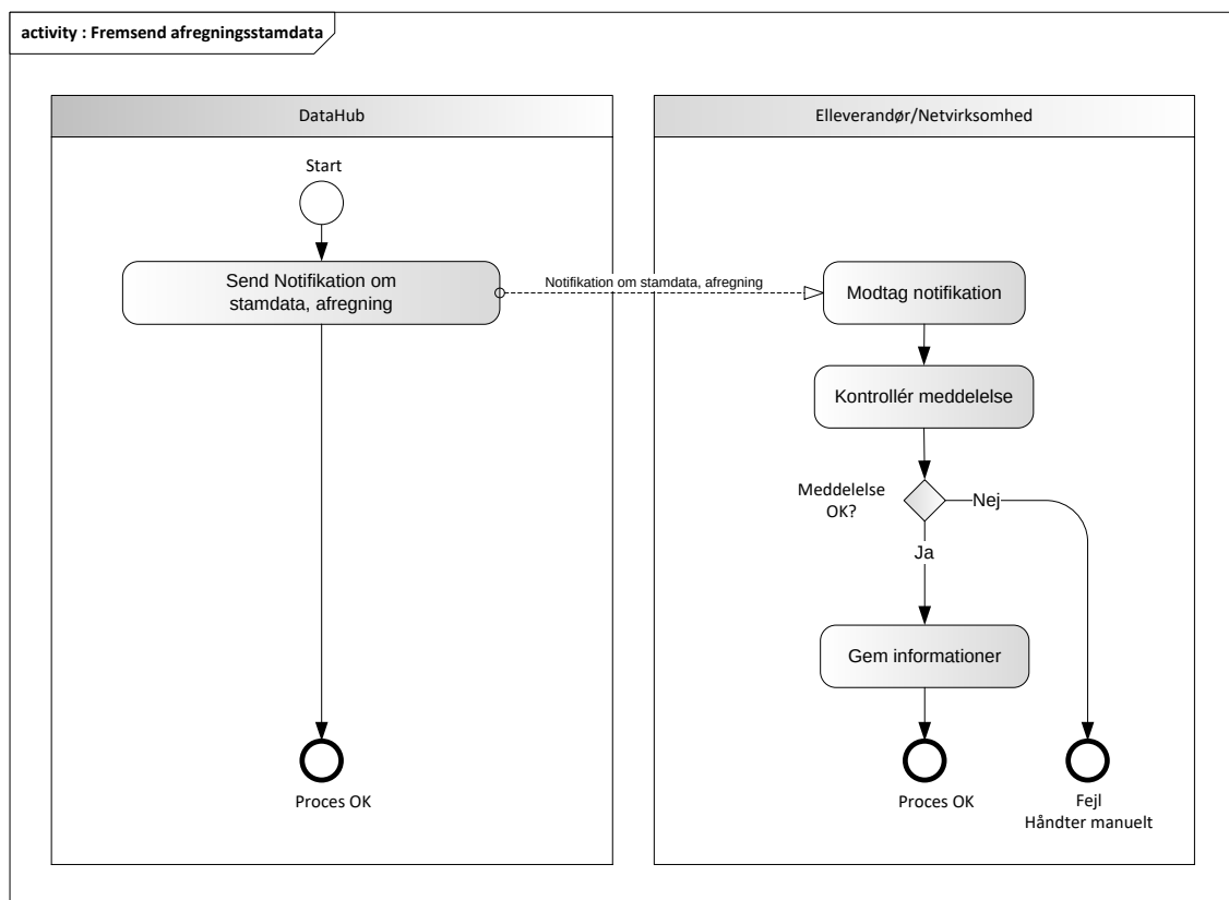
Figur 115115 - Aktivitetsdiagram for Fremsend afregningsstamdata
