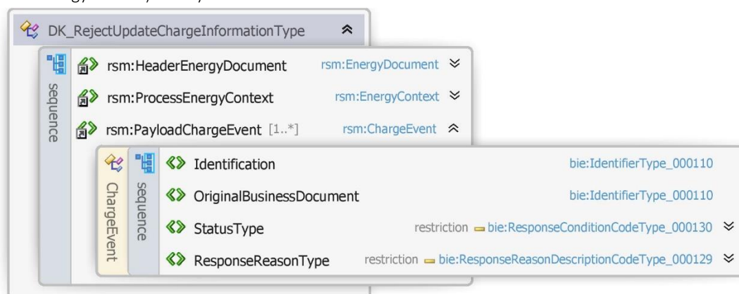
Figur 126126 - Klassediagram for Afvis opdater prislise
