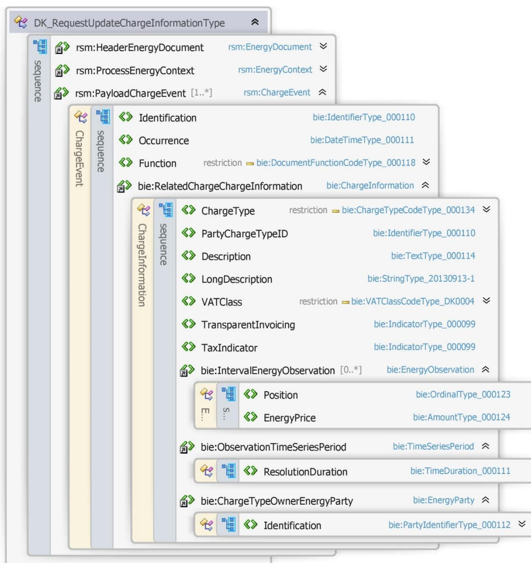
Figur 124124 - Klassediagram for Anmod opdater prislister
