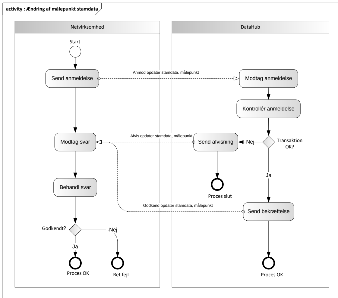
Figur 8080 - Aktivitetsdiagram for Ændring af målepunkt stamdata
