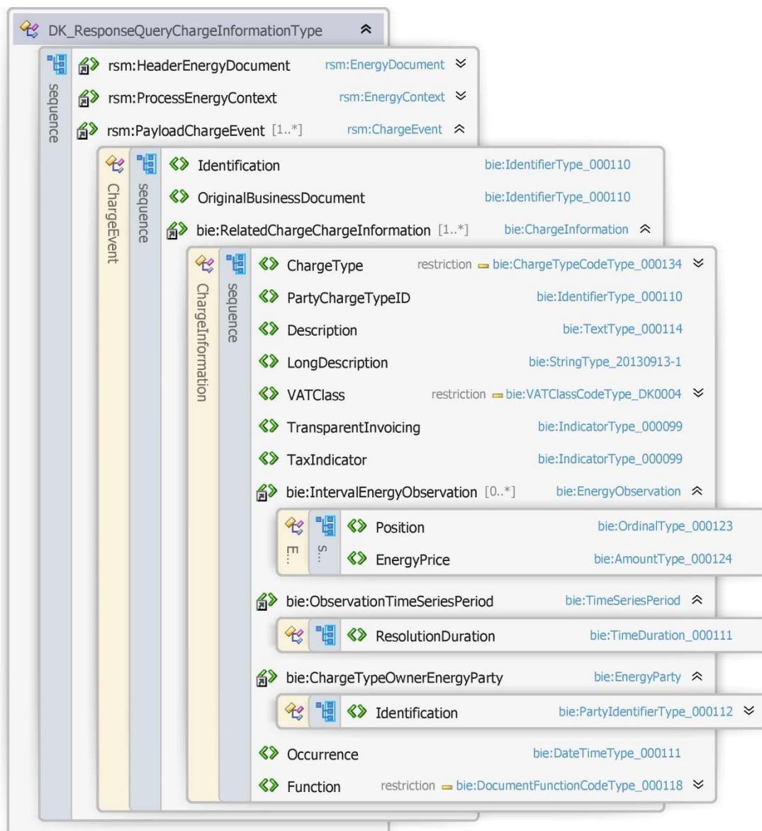
Figur 133133 - Klassediagram for Svar forespørg om prislister
