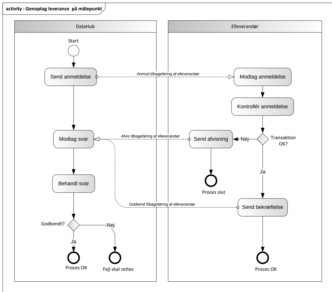
Figur 2020 - Aktivitetsdiagram for Genoptag leverance på målepunkt
