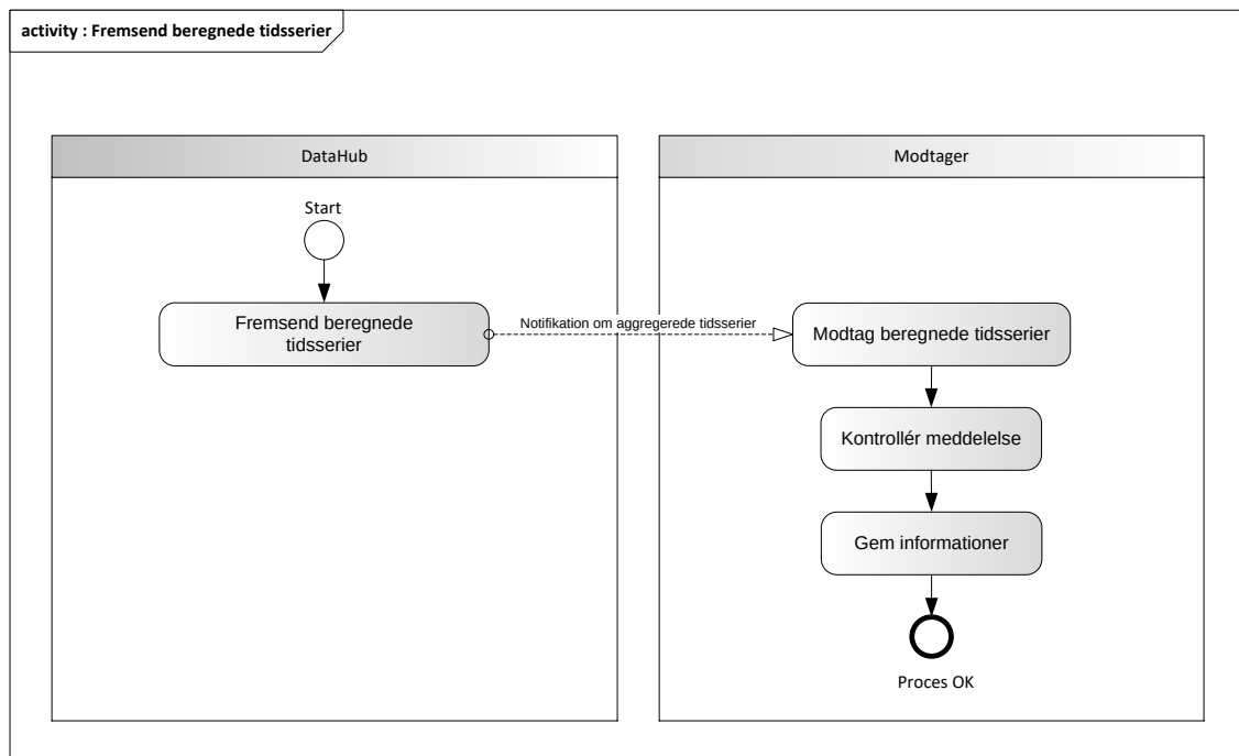
Figur 5454 - Aktivitetsdiagram for Fremsend beregnede tidsserier
