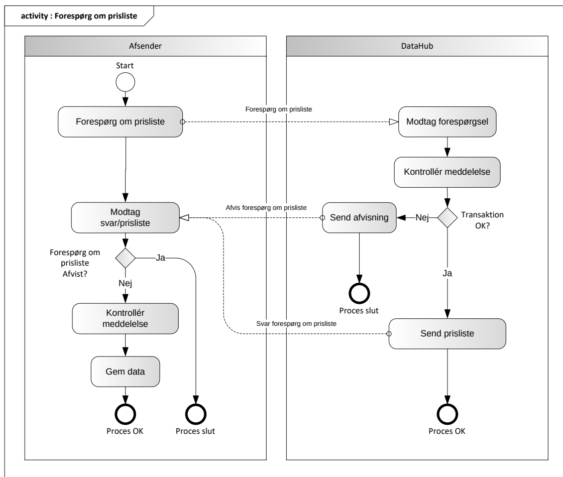
Figur 131131 - Aktivitetsdiagram for forespørg om prisliste
