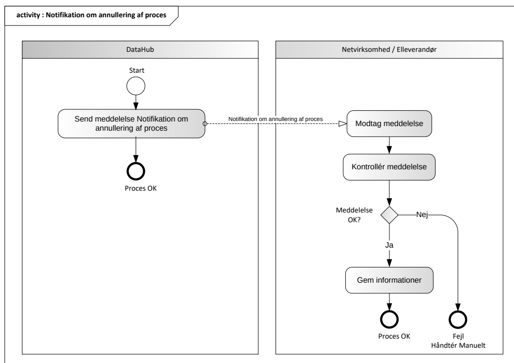
Figur 9696 - Aktivitetsdiagram for Notifikation om annullering
