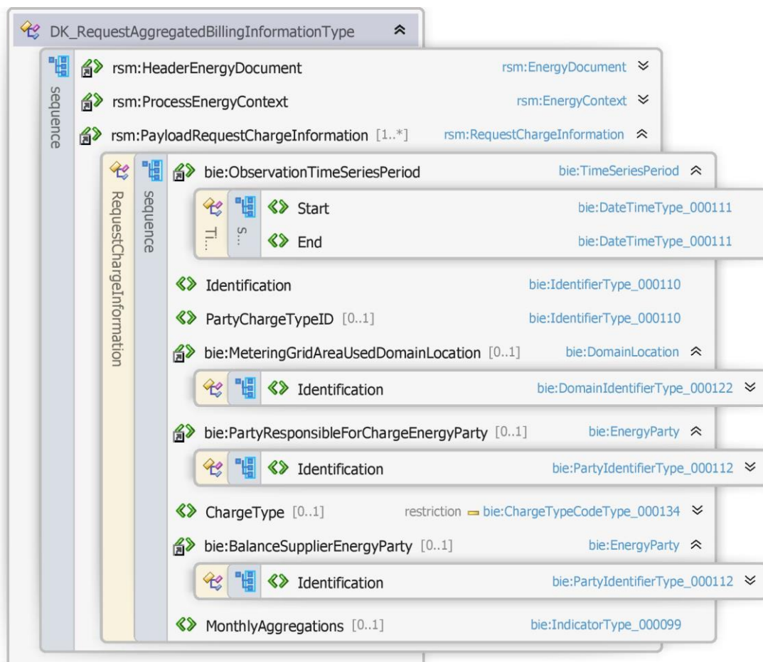
Figur 6666 - Klassediagram for Anmod om engrosydelser
