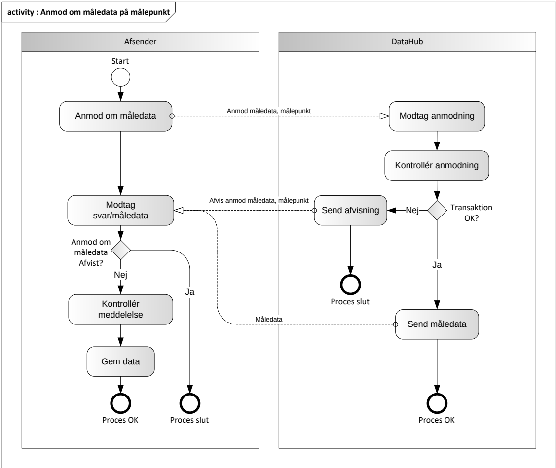
Figur 5757 - Aktivitetsdiagram for Anmod om måledata på målepunkt
