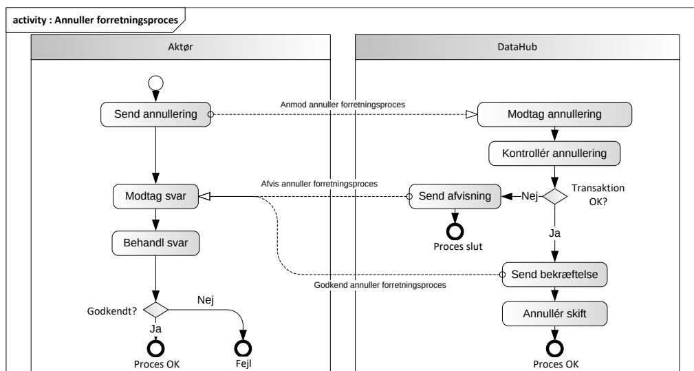
Figur 9191 - Aktivitetsdiagram for Annullering af anmodning
