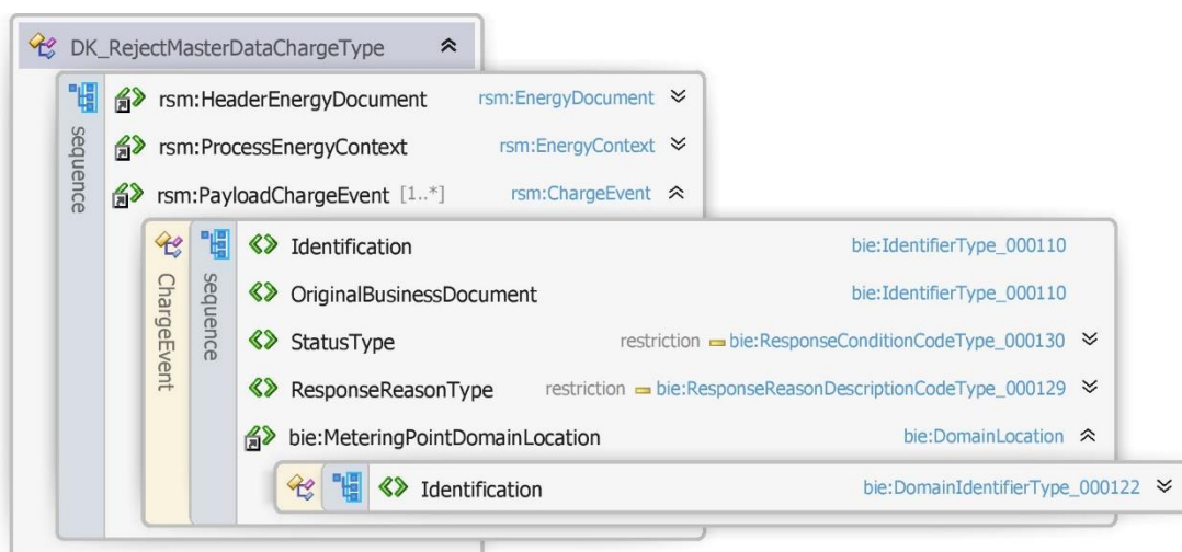
Figur 121121 - Klassediagram for afvis forespørg stamdata, afregning
