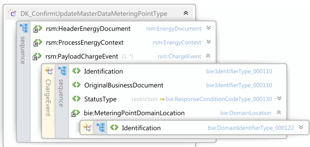
Figur 8282 - Klassediagram for Godkend opdater stamdata, målepunkt
