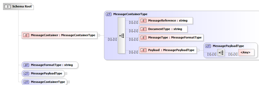
Figur 138138 XML-Beskedstruktur
