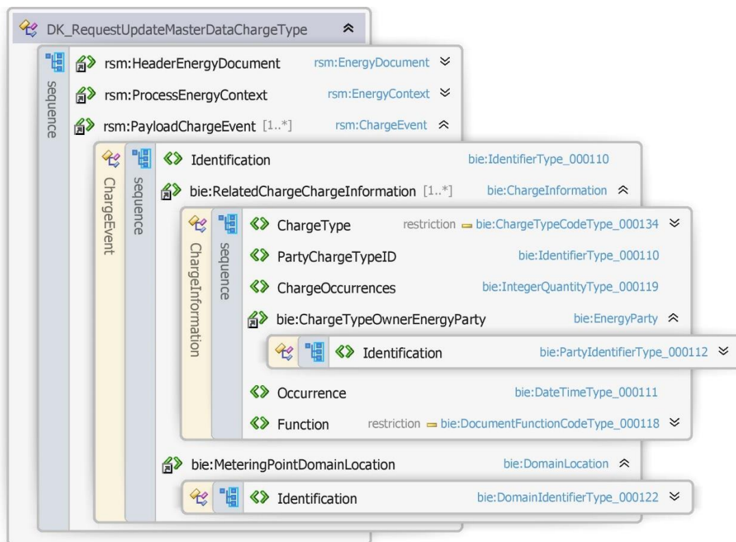
Figur 111111 - Klassediagram for Anmod opdater stamdata, afregning
