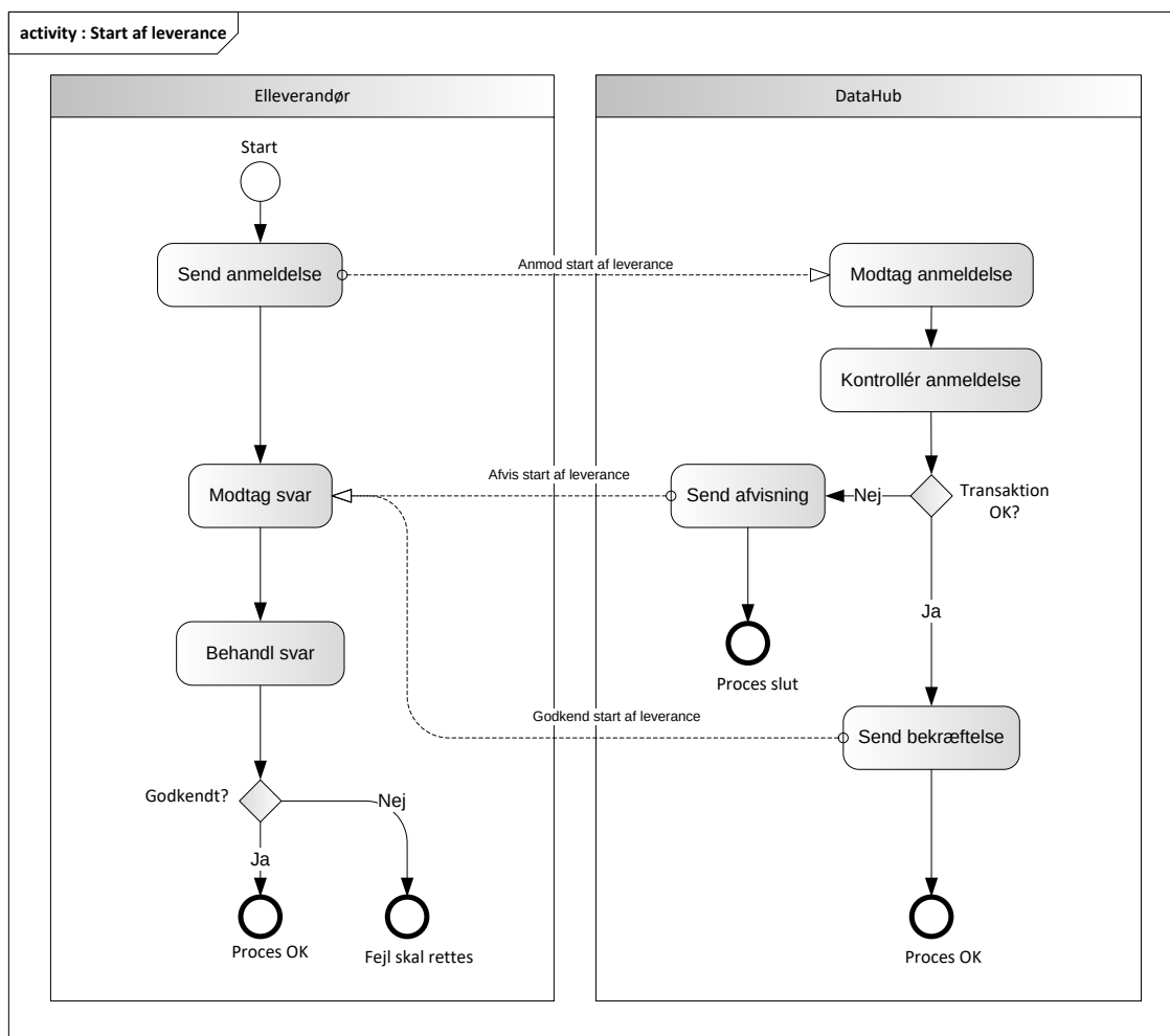
Figur 1010 - Aktivitetsdiagram for Start af leverance
