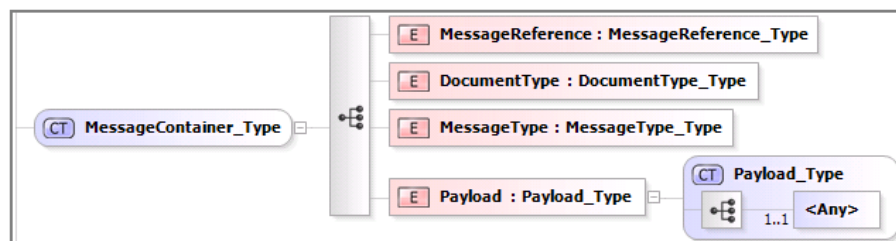
Figur 139139 – XMLSchema, MessageContainer_Type
