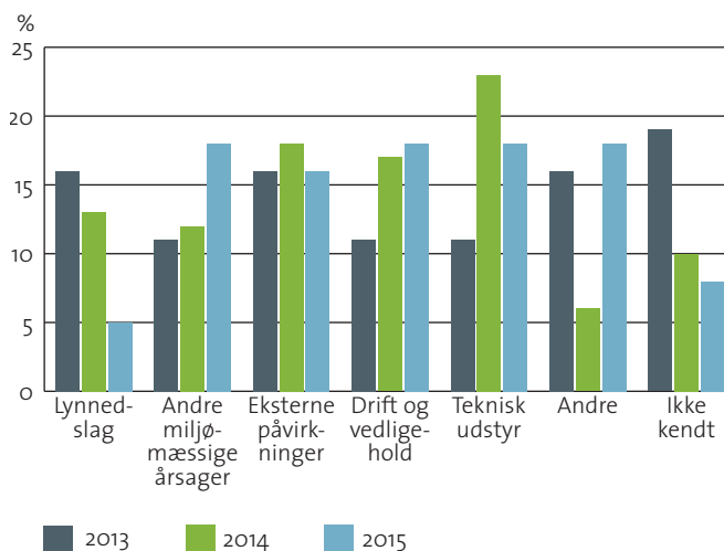
Figur 7. Illustration af den procentvise fordeling af fejl i vekselstrømsnettet (HVAC), Kilde: DISTAC, Nordic and Baltic grid disturbance statistics 2014.
