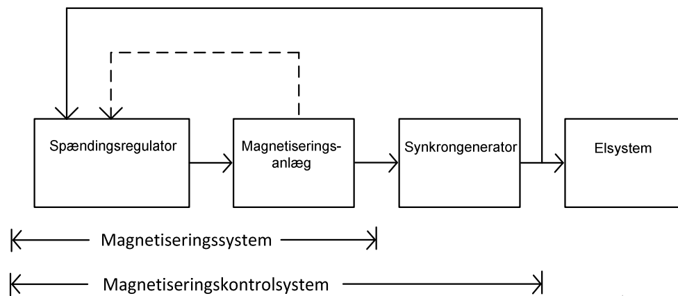
Figur 2 Magnetiseringssystem
