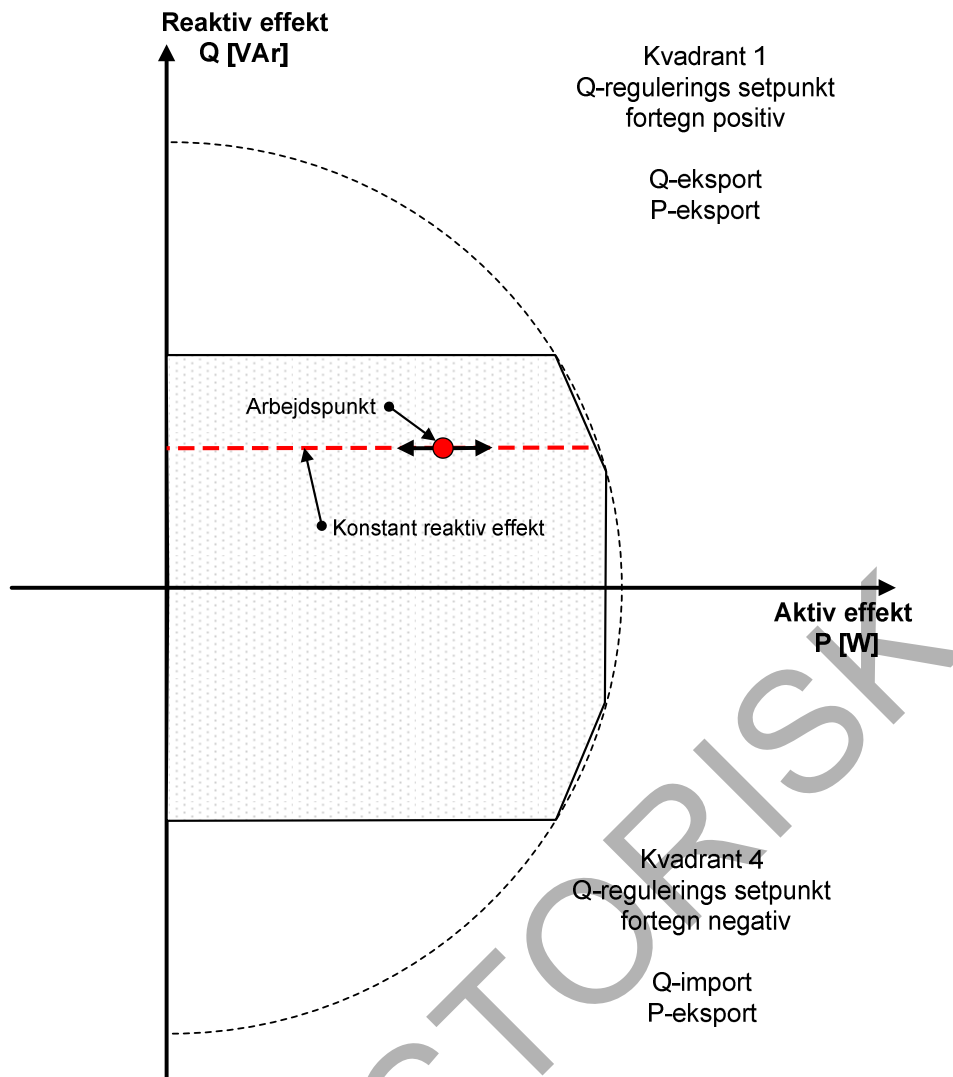
Figur 12 Reaktiv effektreguleringsfunktion for et anlæg (Q-regulering).
