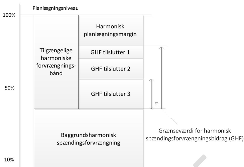
Figur 2 Illustration af metode benyttet til fastsættelse af grænseværdi for harmonisk spændingsforvrængningsbidrag
