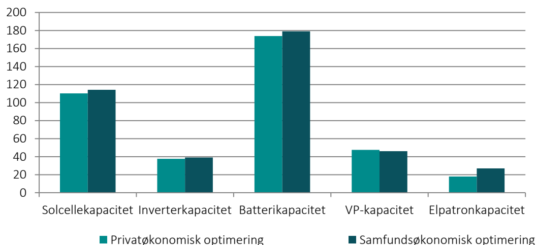
Figur 10 Resultatet af hhv. den privatøkonomiske og samfundsøkonomiske investeringsoptimering i delscenarierne med varmepumper, Forbrugsfleksibilitet med nethensyn og det lave afgiftsniveau. *Batterikapacitet er angivet i kWh, og de resterende elementer i kW.
