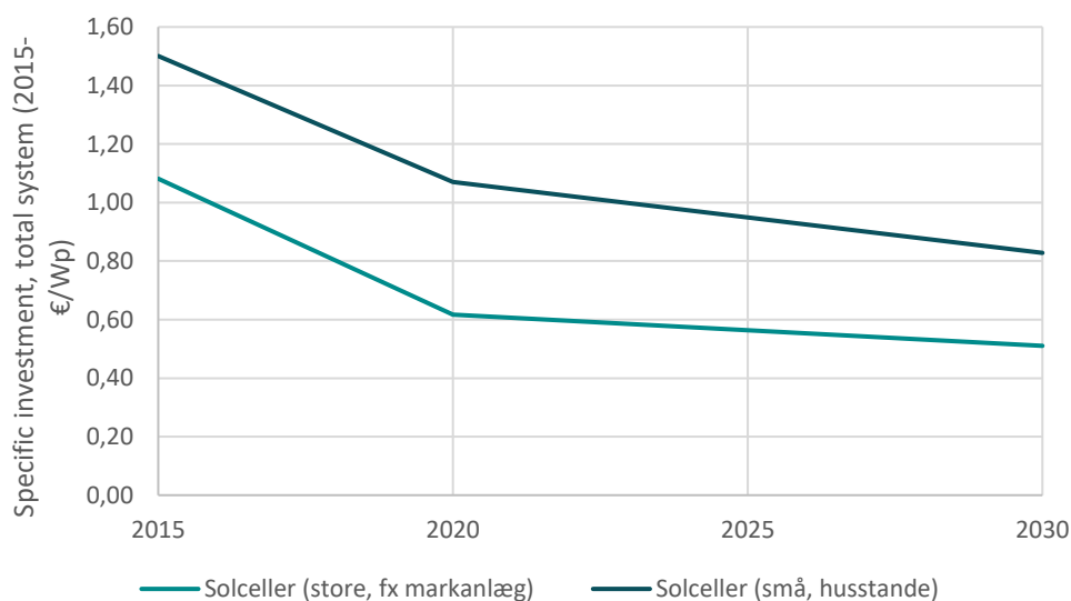
Figur 29. Investeringspriser for små og store solcelleanlæg – forventet fortsat storskala-gevinst ved store anlæg (kilde: Technology Data for Energy storage, Energistyrelsen, 2018)
