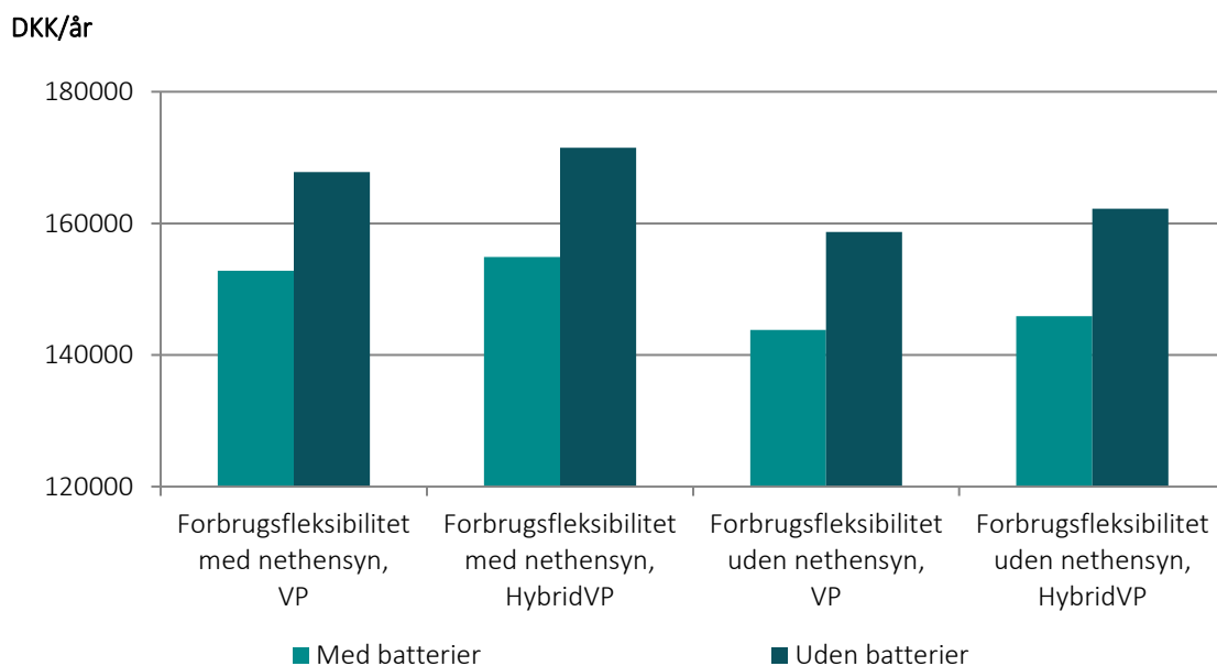
Figur 17 Samlet årlige omkostninger for villavejen i det variationsscenariet uden batterier sammenholdt med referencescenariet (med batterier)
