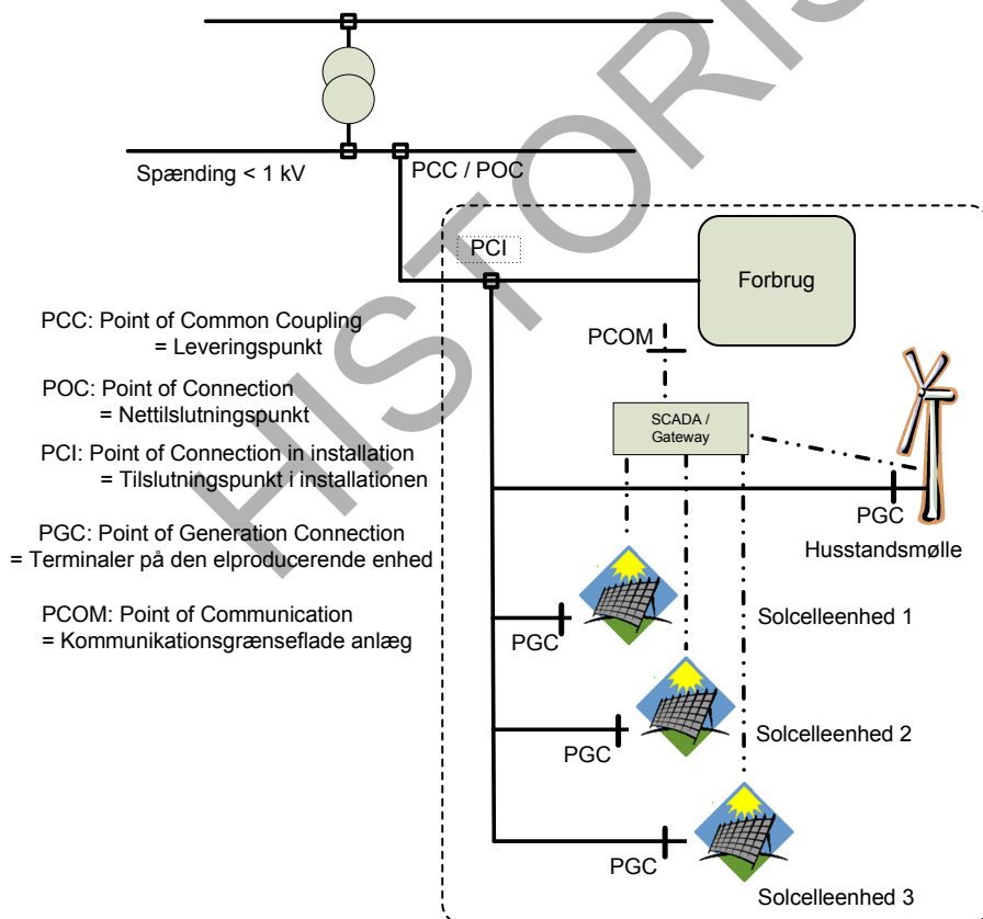
Figur 2 Eksempel på installationstilslutning af et solcelleanlæg.
