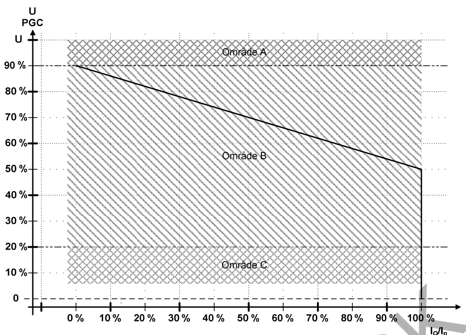
Figur 6 Krav til levering af reaktiv tillægsstrøm I_Q under spændingsdyk for solcelleanlæg kategori C og D.
