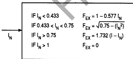
Figur 15 Blokdiagram for ensrettersens reguleringsligning ( F_{EX} = f[I_N] ) for magnetiseringssystemet i figur 13.
