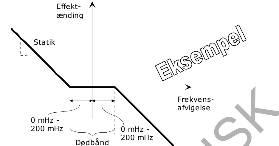
Figur 11 Skitse af indstilling af effekt-/frekvensregulatorens dødbånd.
