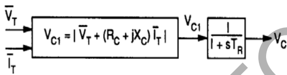
Figur 14 Eksempel på detaljeringsgrad for blokdiagram for transducer til måling af generatorklemspænding for magnetiseringssystemet i figur 13.
