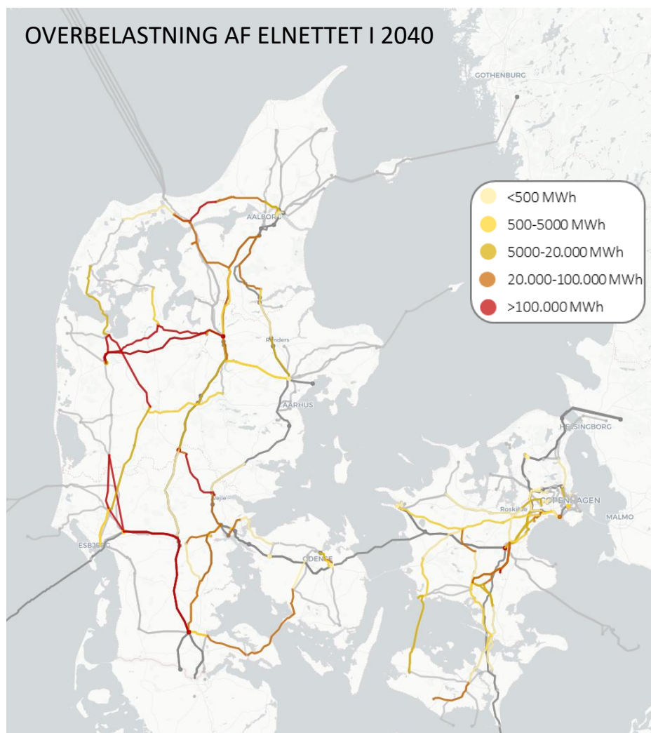
Figur 2 Kortet viser overbelastningsenergien på komponenterne i eltransmissionsnettet som følge af udviklingen i AF20. Opgørelsen er udarbejdet på baggrund af det eksisterende net og projekter, der er godkendt til etablering hos Energinet og myndigheder pr. juni 2021. Overbelastningsenergien angiver den energimængde, der skal aflastes på en forbindelse, hvis ikke der tages andre tiltag i brug. Kritikaliteten af et behov afhænger, ud over størrelsen, af hvad der udløser det (fx forbrug eller produktion) samt omkostningerne forbundet med at afhjælpe det. For mere information om overbelastninger og begreber – se Behovsanalyse for el.
