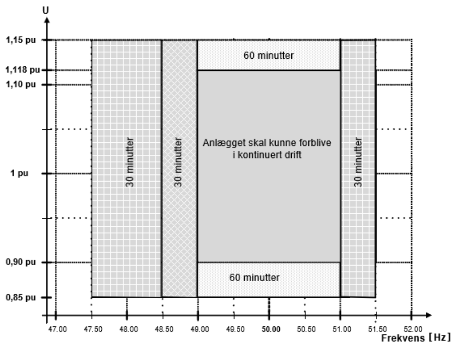
Figur 10 Normaldriftsområde for frekvenser og spændinger ved tilslutning mellem 110-300 kV i DK1.
