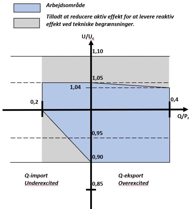
Figur 21 Arbejdsområde for U/U_c .
