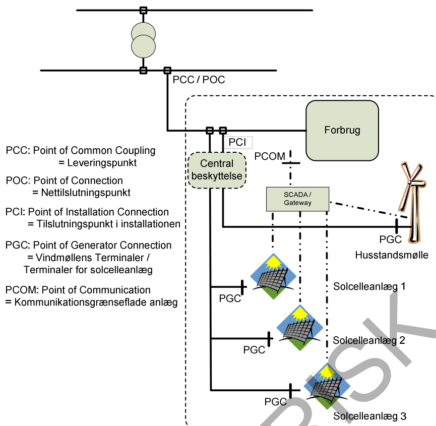
Figur 2 Typisk installationstilslutning af en husstandsmølle.
