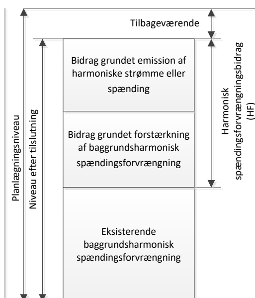
Figur 1 Grafisk præsentation af bidragene til den harmoniske spændingsforvrængning i tilslutningspunktet efter idriftsættelse af anlægget
