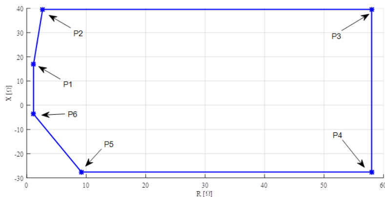
Figur 3 Eksempel på netimpedanspolygon beskrivende for netimpedansen i tilslutningspunktet for anlægget
