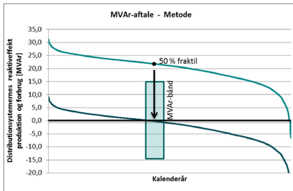
Figur 1: MVar-grænser illustreret sammen med årsvarighedskurven og 50 %-fraktilen.
