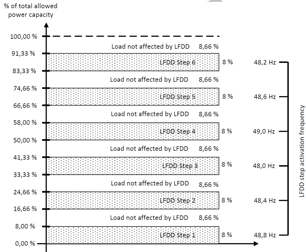
Figur 1: Automatisk LFDD design for kategori 4 — Forbrugsanlæg — Kontinental Europa
