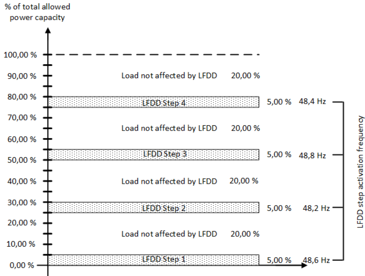
Figur 2: Automatisk LFDD design for kategori 4 - Forbrugsanlæg - Norden
