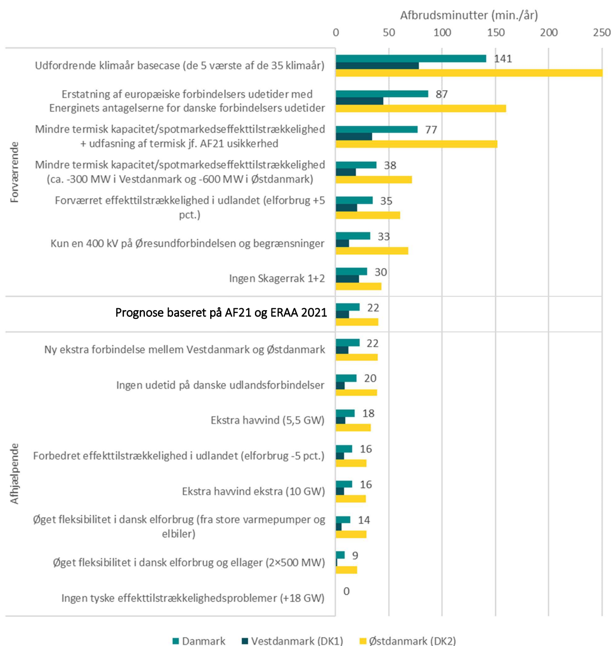
Figur 23 Estimerede afbrudsminutter på grund af manglende effektilstrækkelighed i 2032 i prognose (basisscenarie) og følsomheder.
