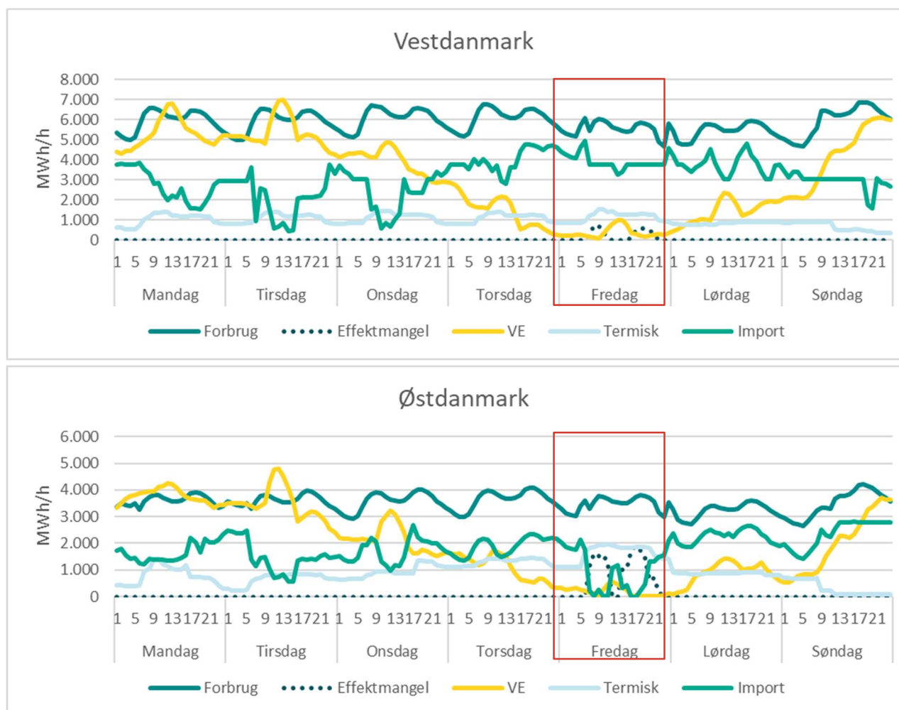
Figur 22 Udvalgt uge i klimaåret 1985 hvor der i en "dunkelflaute" opstår effektilstrækkelighedsproblemer i både Vest- og Østdanmark i 2032. Med rød er markeret den dag hvor der er problemer med effektilstrækkeligheden.
