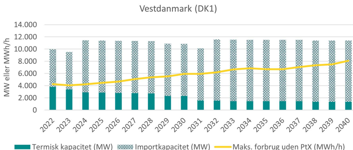
Figur 8 Udvikling for Vestdanmark i AF21. Maks. forbrug er baseret på Energinet modelresultat baseret på AF21 10 og vises uden PtX da dette antages 100 pct. fleksibelt. I effekttilstrækkelighedsberegningerne til Redegørelsen for elforsyning 2022 er forbindelsen til Nordsø Energiøen først antaget idriftsat fra 2033 sammen med vinden på energiøen efter aftale med Energistyrelsen, hvor AF21 modsat har den idriftsat fra 2032.
