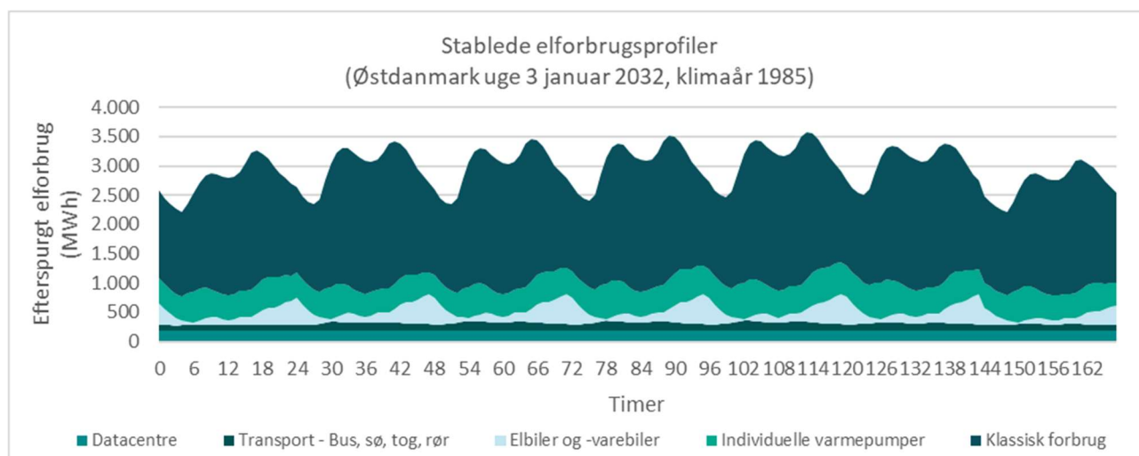
Figur 31 Forbrugsprofiler, som illustreret i figur 30. Stabte elforbrugsprofiler for en effekttilstrækkeligheds-mæssig udfordret uge (mandag til søndag) i januar klimaåret 1985 for året 2032 i Østdanmark (DK2).
