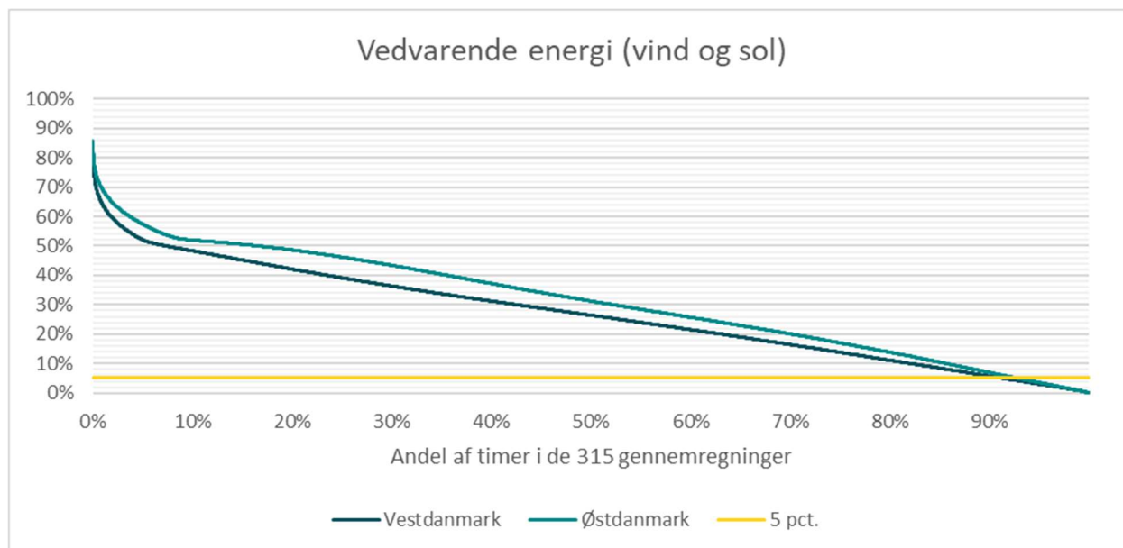
Figur 20 Produktion fra vind og sol sorteret fra højest til lavest i de 315 gennemregninger af 2032 ift. den installerede kapacitet.
