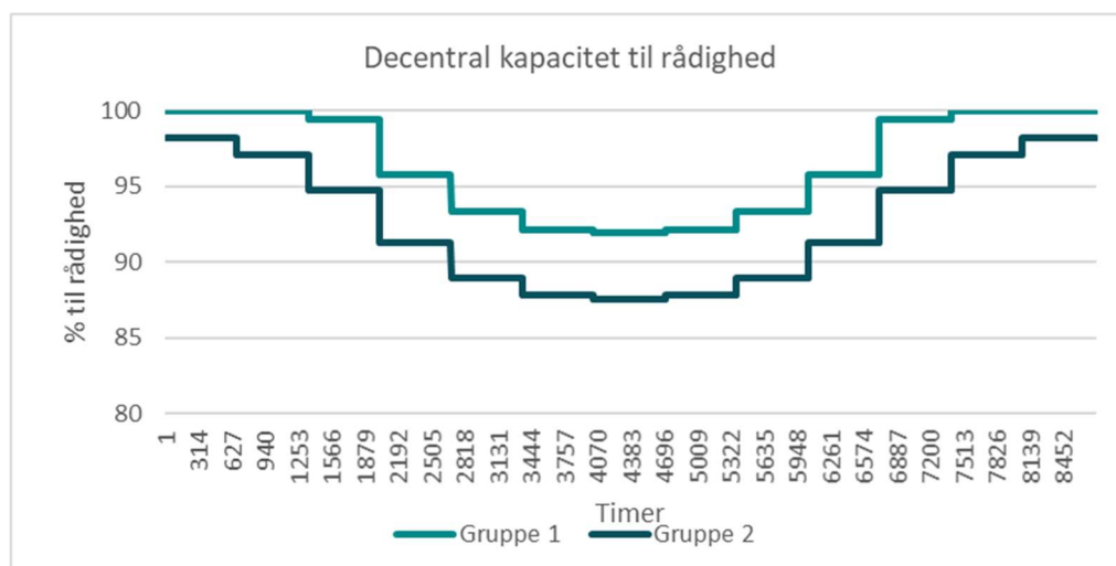
Figur 38 Tilgængelighedsprofilerne for decentral kapacitet. Gruppering på baggrund af værkstype i Tabel 19. Gruppe 1: Light oil, Gas OCGT old, Gas OCGT new. Gruppe 2: Gas CCGT old 1, Gas CCGT old 2, Hard coal old 1, Heavy oil old 1.
