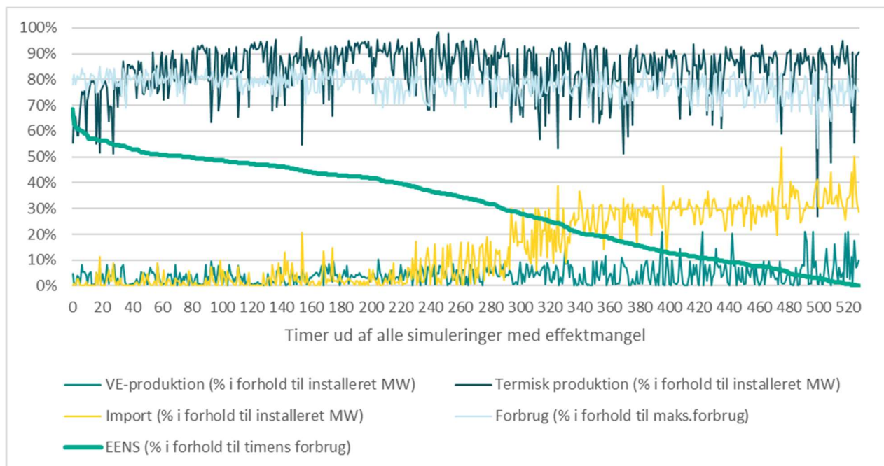
Figur 18 Effektmangelssituationer i Østdanmark i 2032 sorteret efter den største procentvise effektmangel ift. timens elforbrug vist sammen med andelen af henholdsvis VE og termisk produktion, samt import og forbrug i forhold til deres maksimale værdier. Figuren viser kun de 528 timer med effektilstrækkelighedsproblemer ud af alle simulerede timer (315 x 8760). I Østdanmark regnes med 7.675 MW installeret VE, 2.059 MW termisk effekt, 4.390 MW importkapacitet og et maksimalforbrug på 4.650 MWh/h på tværs af alle klimaaår.
