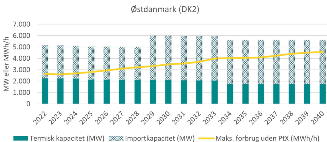
Figur 9 Udvikling for Østdanmark i AF21. Maks. forbrug er baseret på Energinet modelresultat baseret på AF21 11 og vises uden PtX da dette antages 100 pct. fleksibelt.
