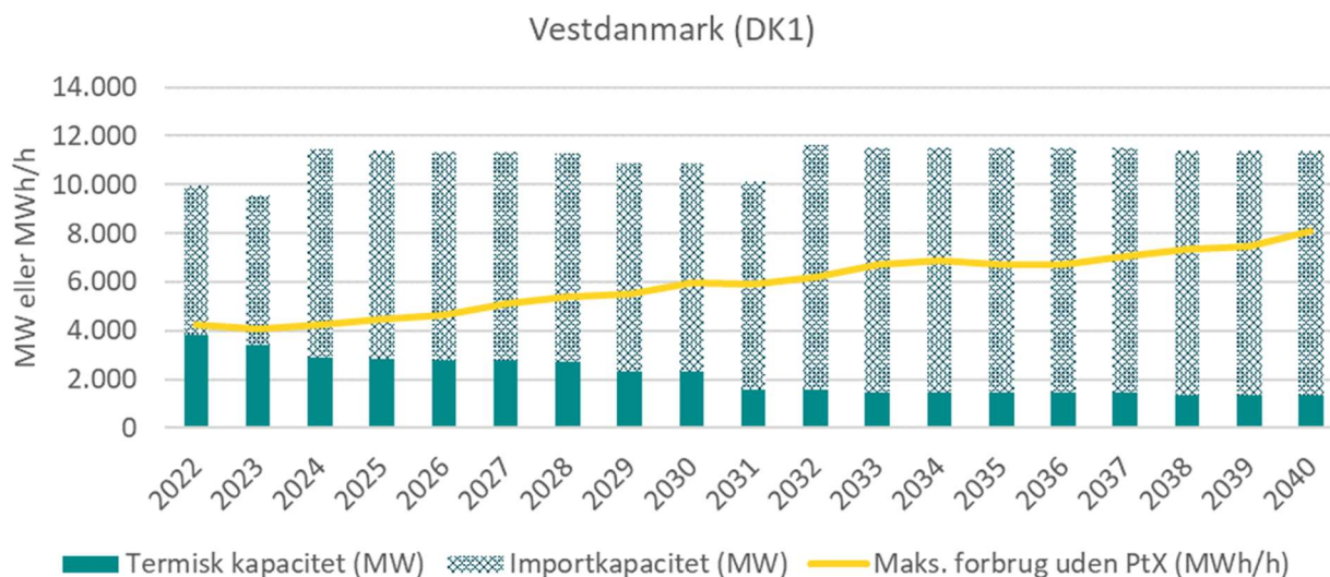
Figur 8 Udvikling for Vestdanmark i AF21. Maks. forbrug er baseret på Energinets modelresultat baseret på AF21 11 og vises uden PtX, da dette antages 100 pct. prisfleksibelt. I effekttilstrækkelighedsberegningerne til Redegørelsen for elforsyning 2022 er forbindelsen til Nordsø Energiøen først antaget idriftsat fra 2033 sammen med vinden på energiøen efter aftale med Energistyrelsen, hvor AF21 modsat har den idriftsat fra 2032.
