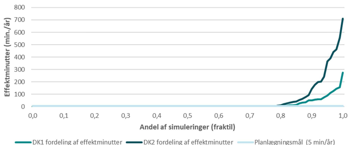
Figur 6 Fordeling af effektminutter (= afbrudsminutter relateret til effekttilstrækkelighed) i 2032-prognosen på tværs af de 315 simuleringsår der består af 35 klimaår som gennemkøres 9 gange hver med forskellige stokastiske havarimønstre. I nedenstående boks uddybes karakteristika og størrelse for timerne med effektmangel.
