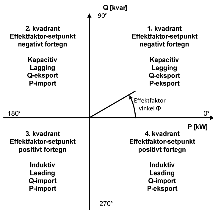
Figur 1 Definition af fortegn for aktiv effekt, reaktiv effekt, effektfactor-setpunkter samt reference for effektfactorvinkel.
