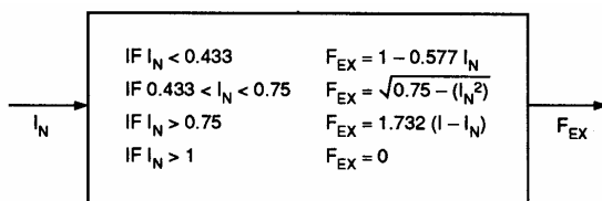
Figur 13 Blokdiagram for ensretterens reguleringsligning ( F_{EX} = f[I_N] ) for magnetiseringsystemet i figur 11.
