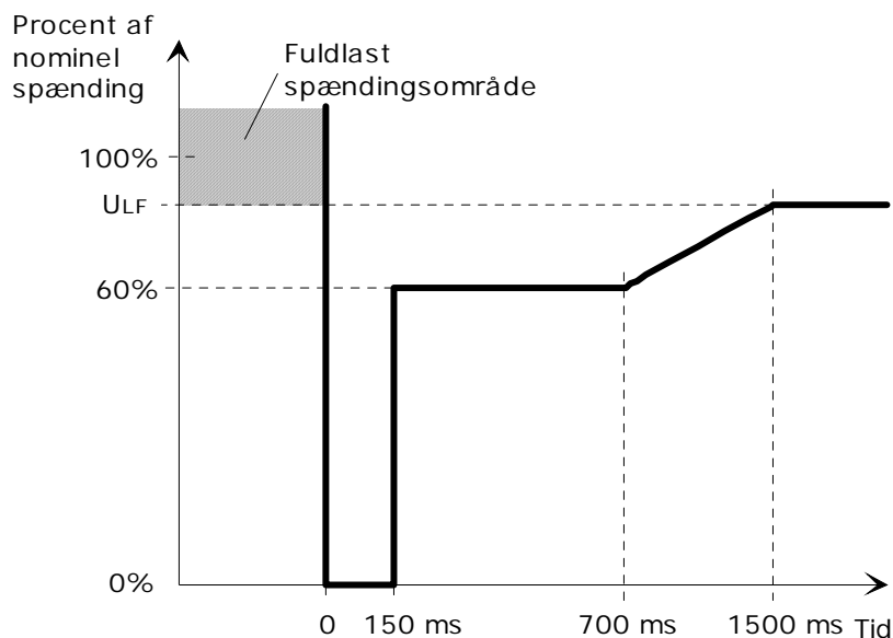
Figur 1 3-faset spændingsforstyrrelse som ikke må lede til udkobling af kraftværksenheden . U_{LF} betegner den nedre grænse for fulldlast spændingsområdet, jf. 5.2.2.
