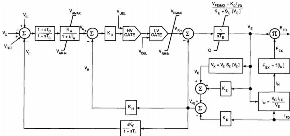
Figur 11 Blokdiagram for et magnetiseringsystem.
