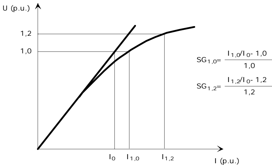
Figur 4 Definition af generatorens mætningspunkter SG_{1,0} og SG_{1,2} ud fra tomgangskararakteristikken.
