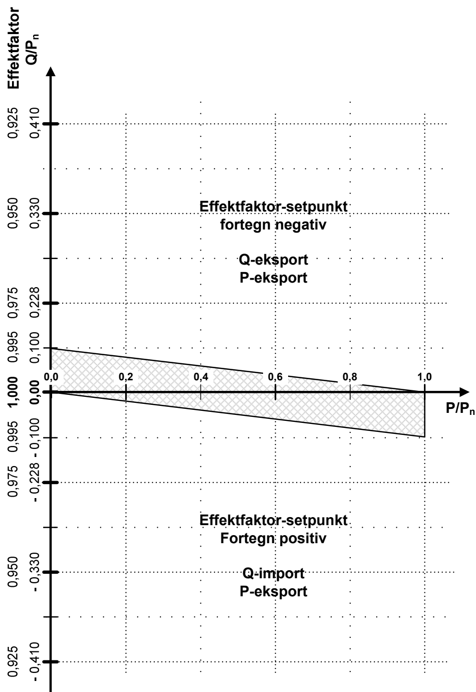
Figur 17 Krav til levering af reaktiv effekt i forhold til aktiv effekt niveau ved U_c for vindkraftværker i kategori B.
