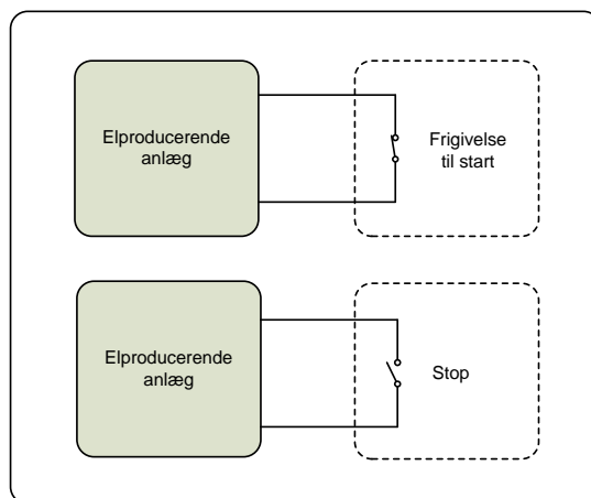
Figur 2 Mulig signaludveksling til eksternt stop og frigivelse til start
