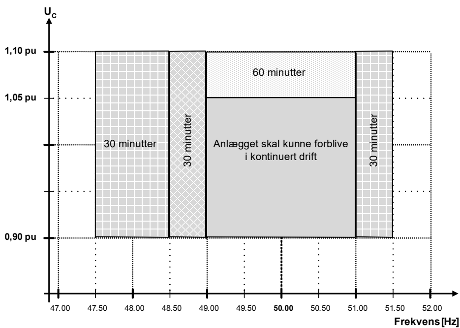
Figur 9 Normaldriftsområde: transmissionstilsluttede anlæg i DK2, 110-300 kV.
