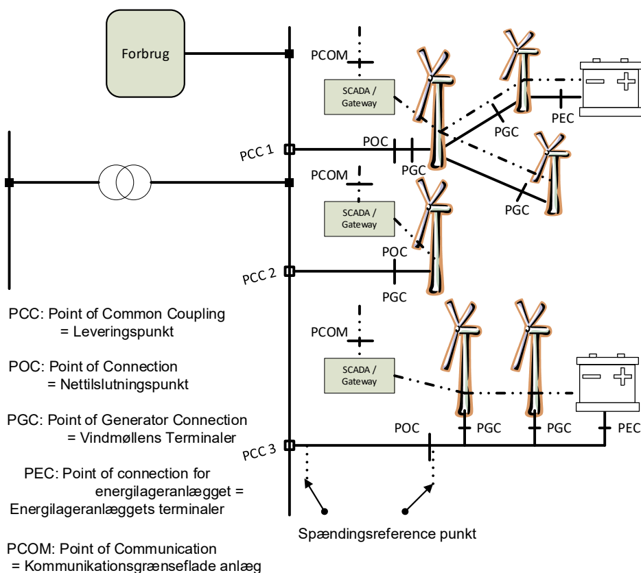
Figur 4 Eksempel på nettilslutning af anlæg.
