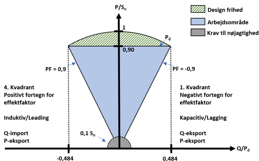
Figur 27 Krav til levering af reaktiv effekt ved arbejds punkter mindre end P_{n1} for energilageranlæg i kategori A og B tilsluttet lavspænding.
