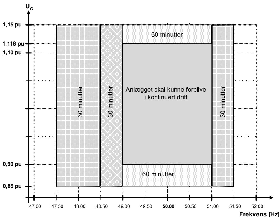
Figur 7 Normaldriftsområde: transmissionstilsluttede anlæg i DK1, 110-300 kV.
