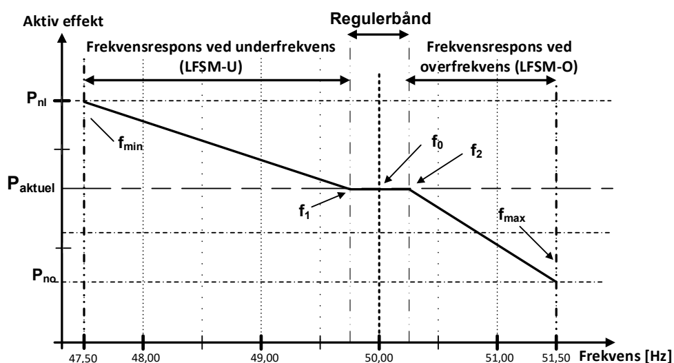
Figur 19 Frekvensrespons fra et energilageranlæg, som kan levere og optage effekt fra det kollektive elforsyningsnet. Figuren anskueliggør funktioner og respons, men værdier foruden frekvensrelaterede værdier er fiktive.
