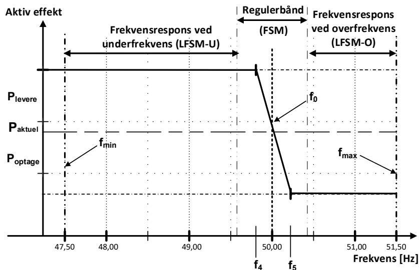
Figur 21 FSM-bånd, FCR-N og frekvensrespons i DK2. Figuren anskueliggør funktioner og respons, men værdier foruden frekvensrelaterede værdier er fiktive.
