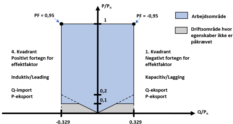
Figur 31 Krav til levering af reaktiv effekt ved arbejds punkter mindre end P_{ni} for energilageranlæg i kategori C.
